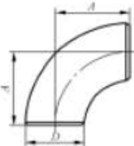
图 4 短半径 90°弯头
