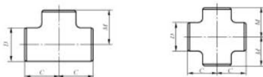
图 7 等径三通和四通
