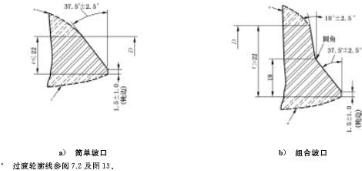
图 12 管件端部坡口形状及尺寸
