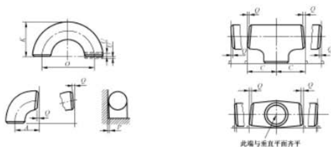
图 14 公差简图
