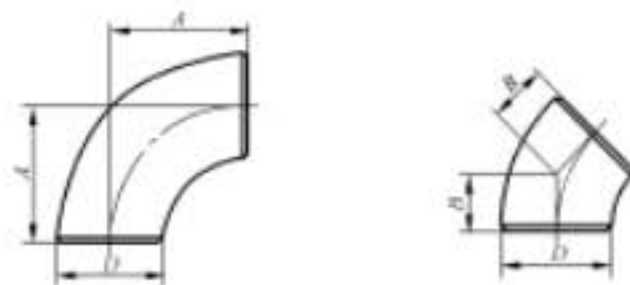
图 1 长半径 90°和 45°弯头
