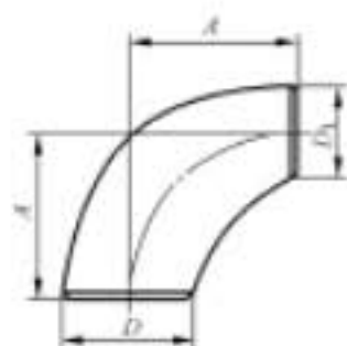
图 2 90°长半径异径弯头
